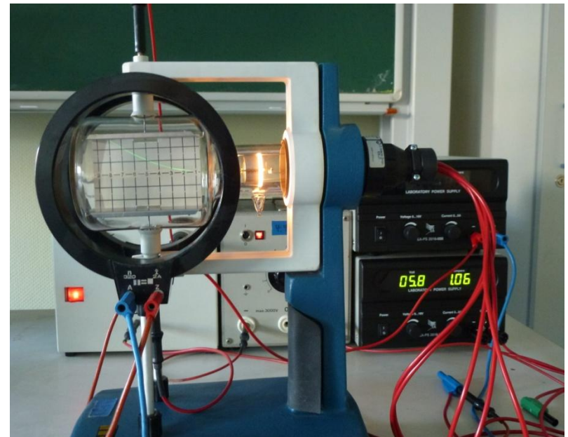
Elektronenstrahlröhre und Fadenstrahlrohr für Physikunterricht
